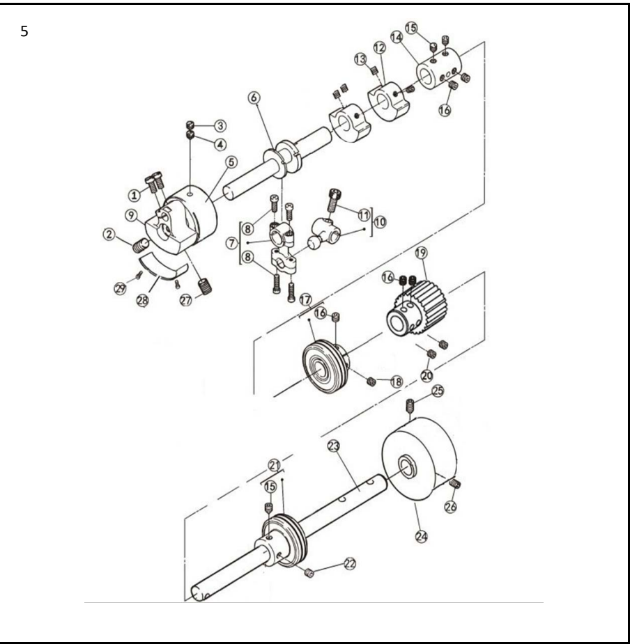
五、上轴部件/Main shaft assembles
