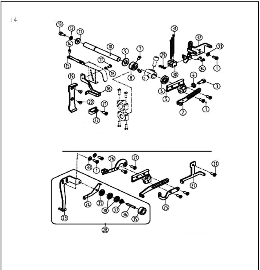
十四、过线部件/Thread loosening assemblies
