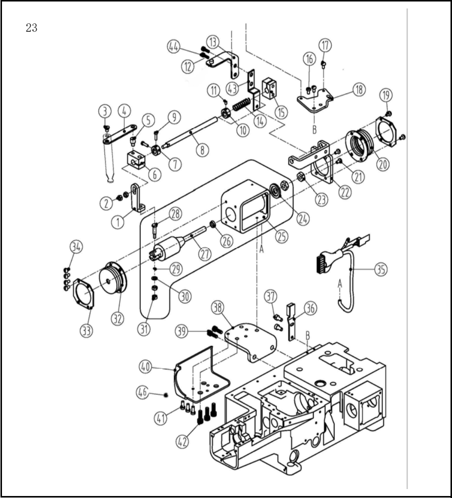
二十三、剪线电磁铁部件/Solenoid assemblies
