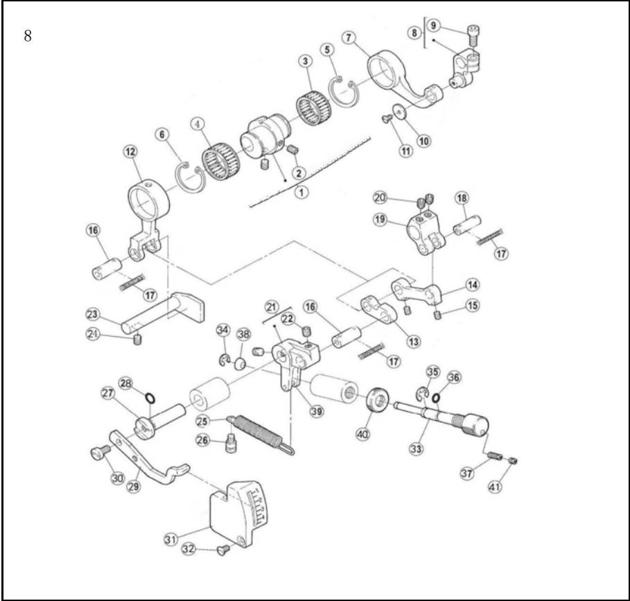
八、护针部件/Feed mechanism
