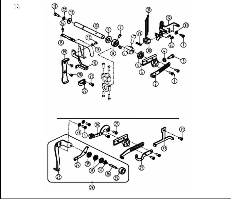
十三、过线部件/Thread loosing assemblies
