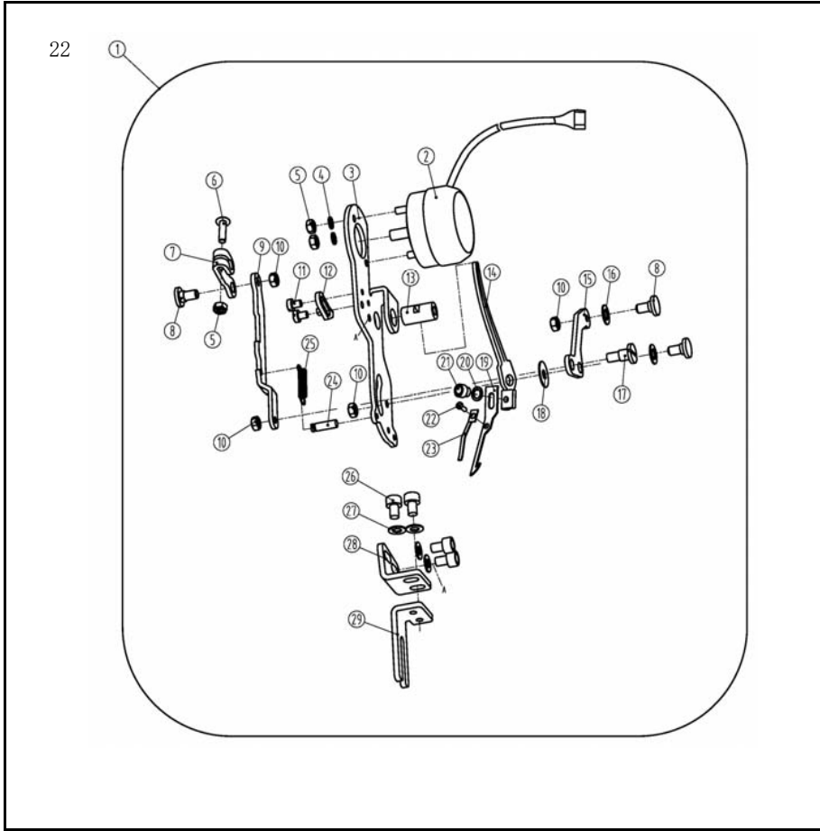
二十二、拨线器部件/Top wiper assemblies
