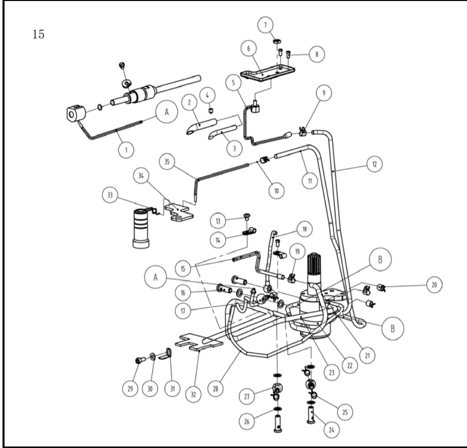
十五、润滑部件/Lubricatrn assemblies
