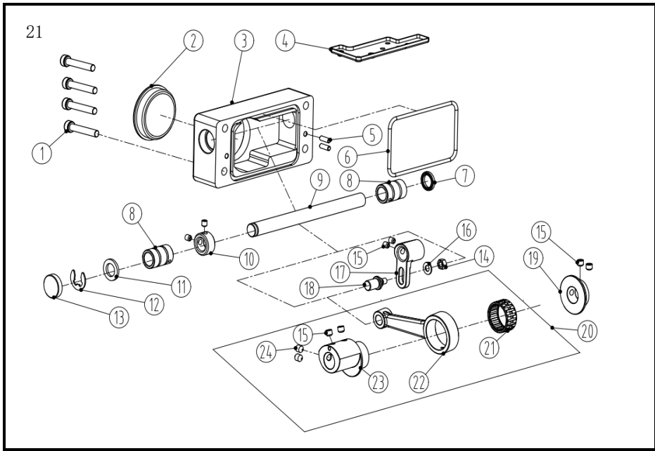
二十一、后拖轮架部件/After fight cam assemblies
