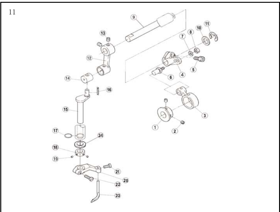
十一、喂针部件/Needle feeding assemblies
