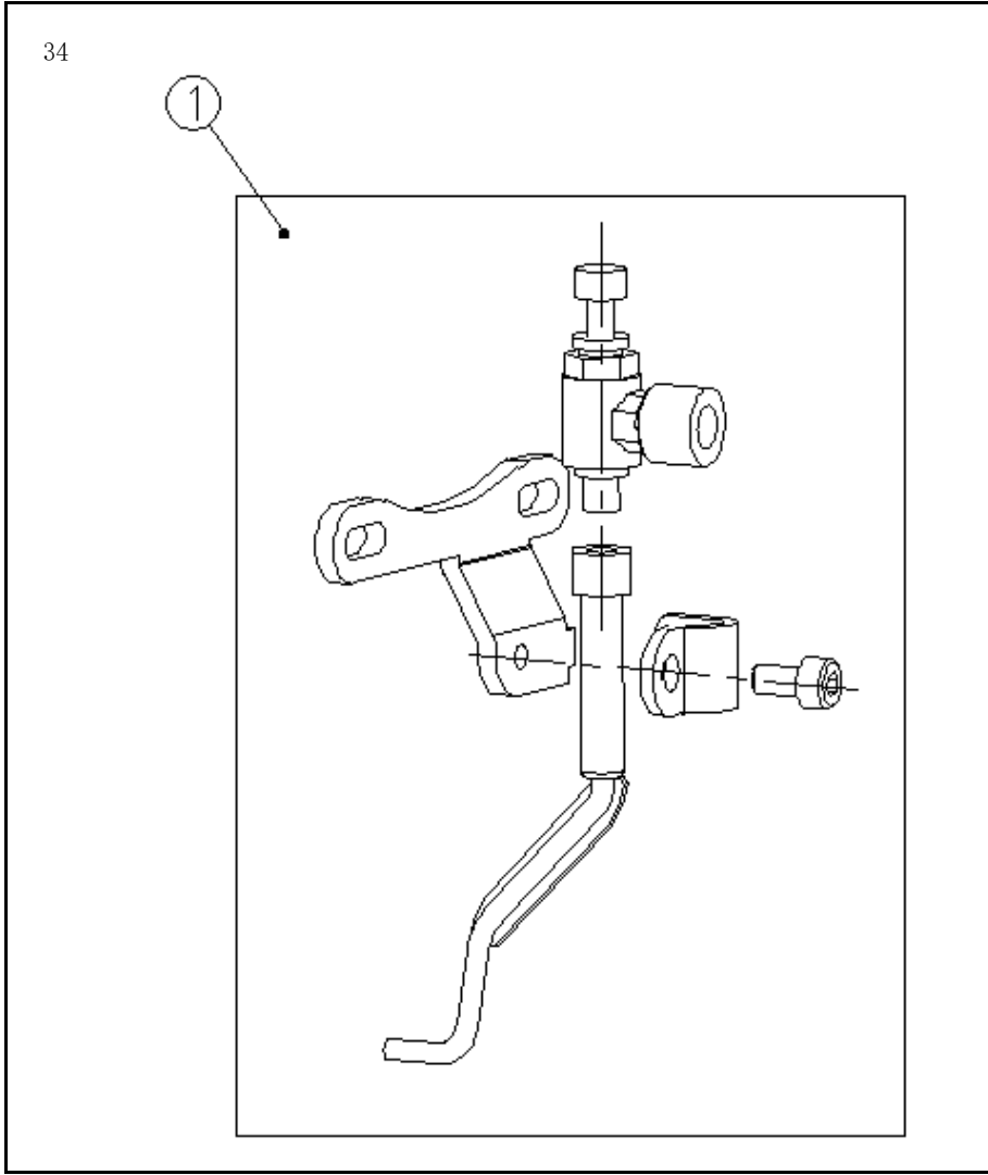
三十四、吹线部件/Blowing unit
