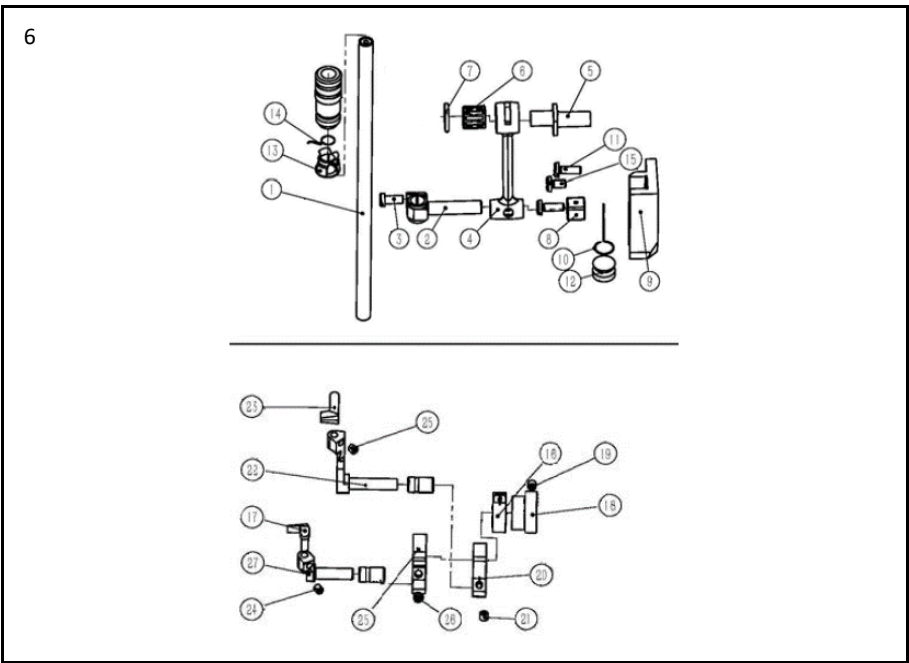
六、针杆部件/Needle bar assemblies
