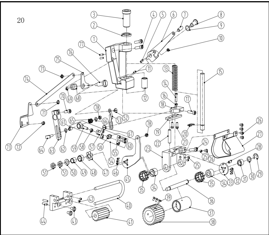
二十、后拖轮部件/After cam assemblies
