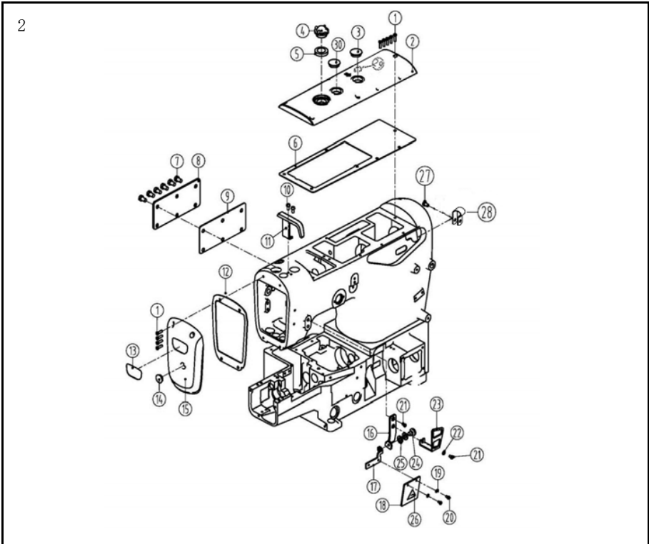
二、罩壳部件/Cover assemblies
