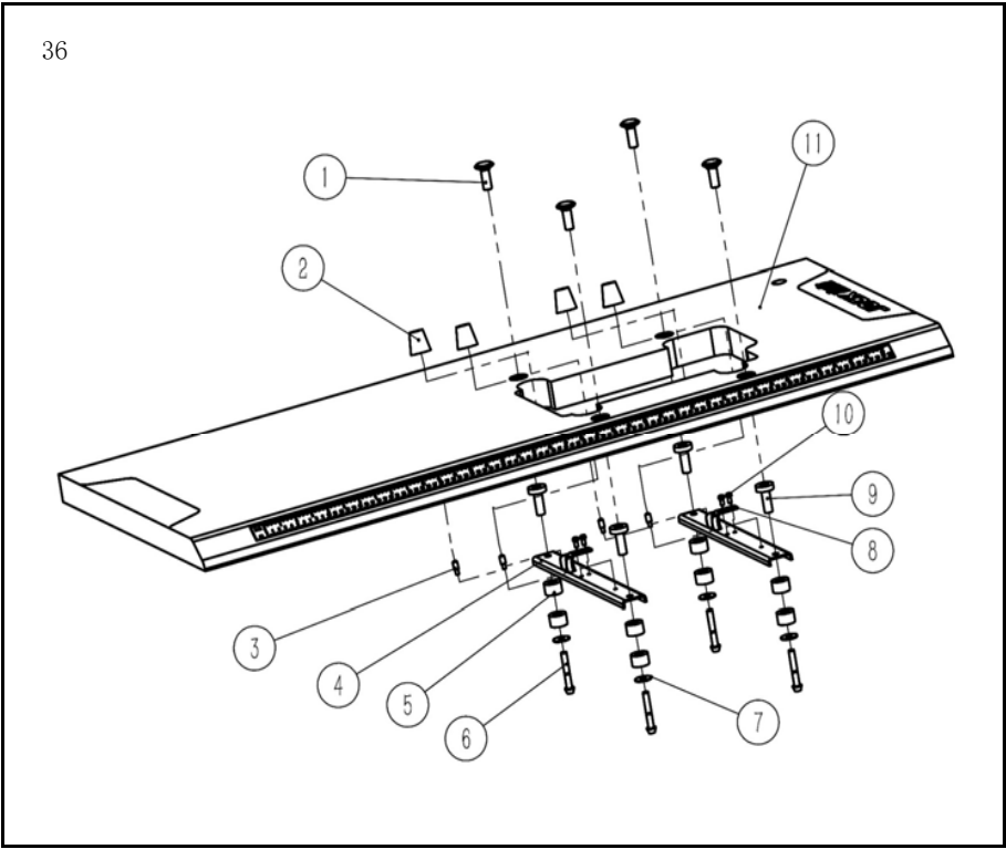
三十六、台板部件/Bedplate assemblies
