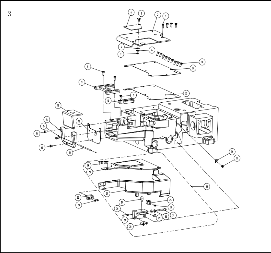
三、缝台部件/Cloth plate assemblies
