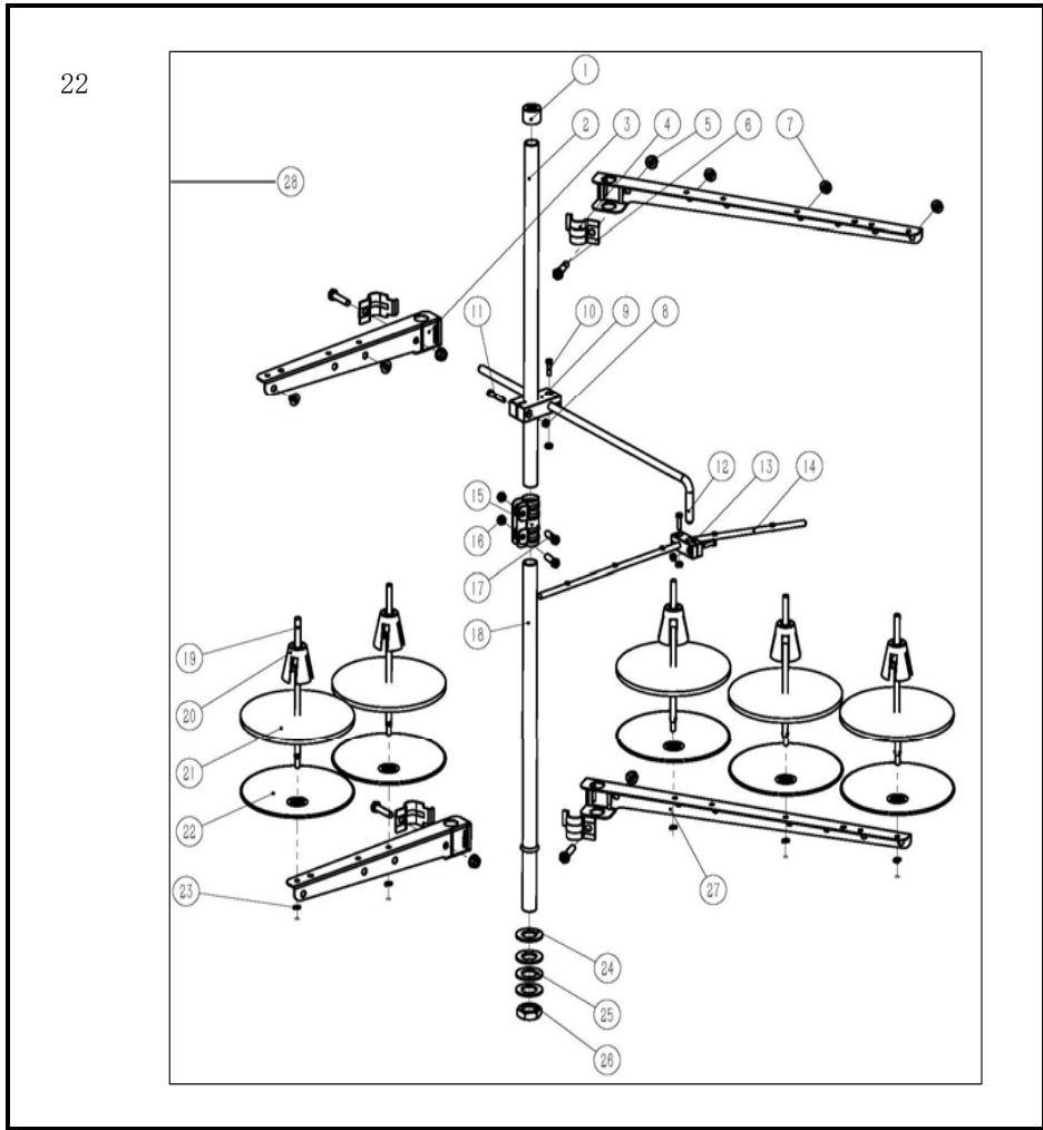
二十二、线架部件/Thread apool assemblies
